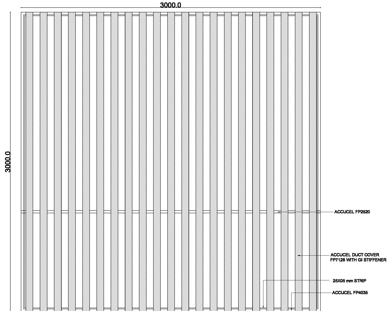
ELEVATION
