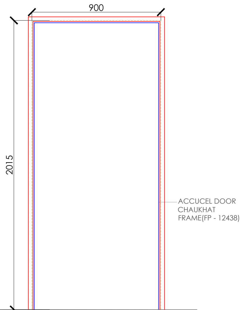
FRAME ELEVATION
